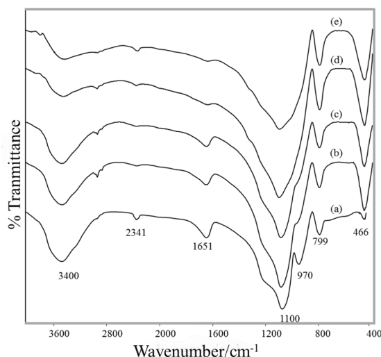
Figure 3. FTIR Spectra of Materials (a) \text{Nb}/\text{SiO}_2\text{-TiO}_2 , (b) 0.05\text{PO}_4^-/\text{Nb}/\text{SiO}_2\text{-TiO}_2 , (c) 0.10\text{PO}_4^-/\text{Nb}/\text{SiO}_2\text{-TiO}_2 , (d) 0.15\text{PO}_4^-/\text{Nb}/\text{SiO}_2\text{-TiO}_2 , (e) 0.20\text{PO}_4^-/\text{Nb}/\text{SiO}_2\text{-TiO}_2
