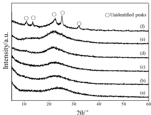
Figure 2. X-Ray Diffractograms of Materials (a) \text{Nb}/\text{SiO}_2\text{-TiO}_2 , (b) 0.05\text{PO}_4^-/\text{Nb}/\text{SiO}_2\text{-TiO}_2 , (c) 0.10\text{PO}_4^-/\text{Nb}/\text{SiO}_2\text{-TiO}_2 , (d) 0.15\text{PO}_4^-/\text{Nb}/\text{SiO}_2\text{-TiO}_2 , (e) 0.20\text{PO}_4^-/\text{Nb}/\text{SiO}_2\text{-TiO}_2 and (f) 0.25\text{PO}_4^-/\text{Nb}/\text{SiO}_2\text{-TiO}_2
